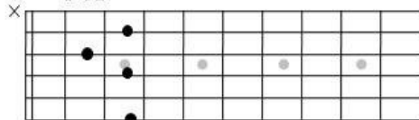
Fm6 /G
